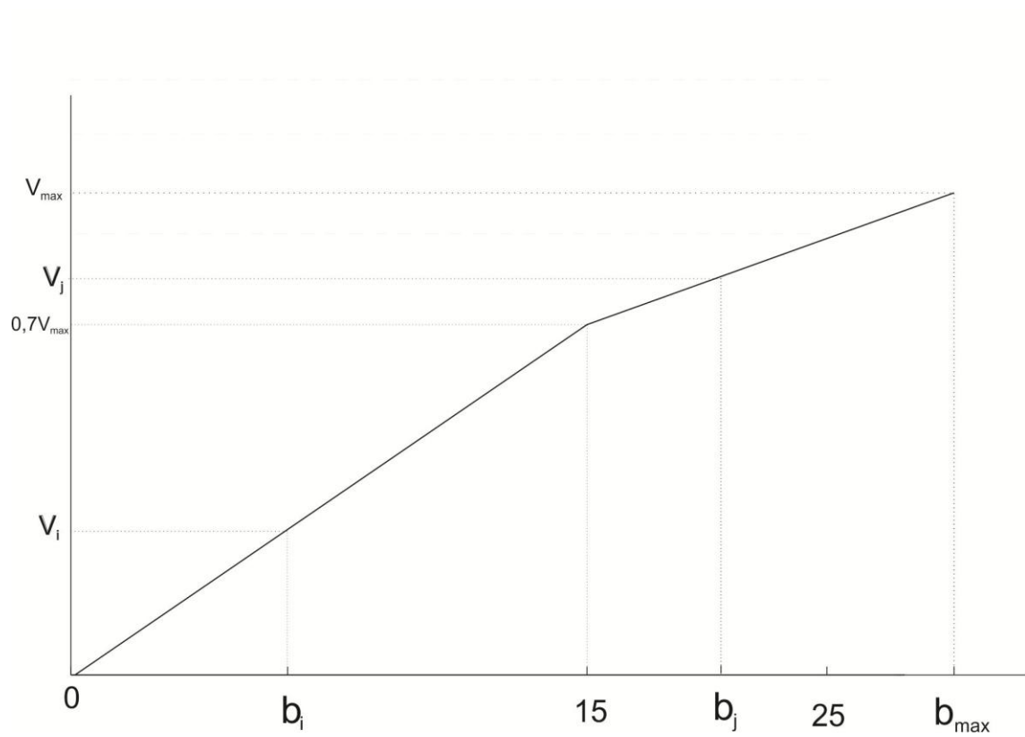
Figura 3: Representación gráfica de las puntuaciones si b_{\max} \geq 25 .
