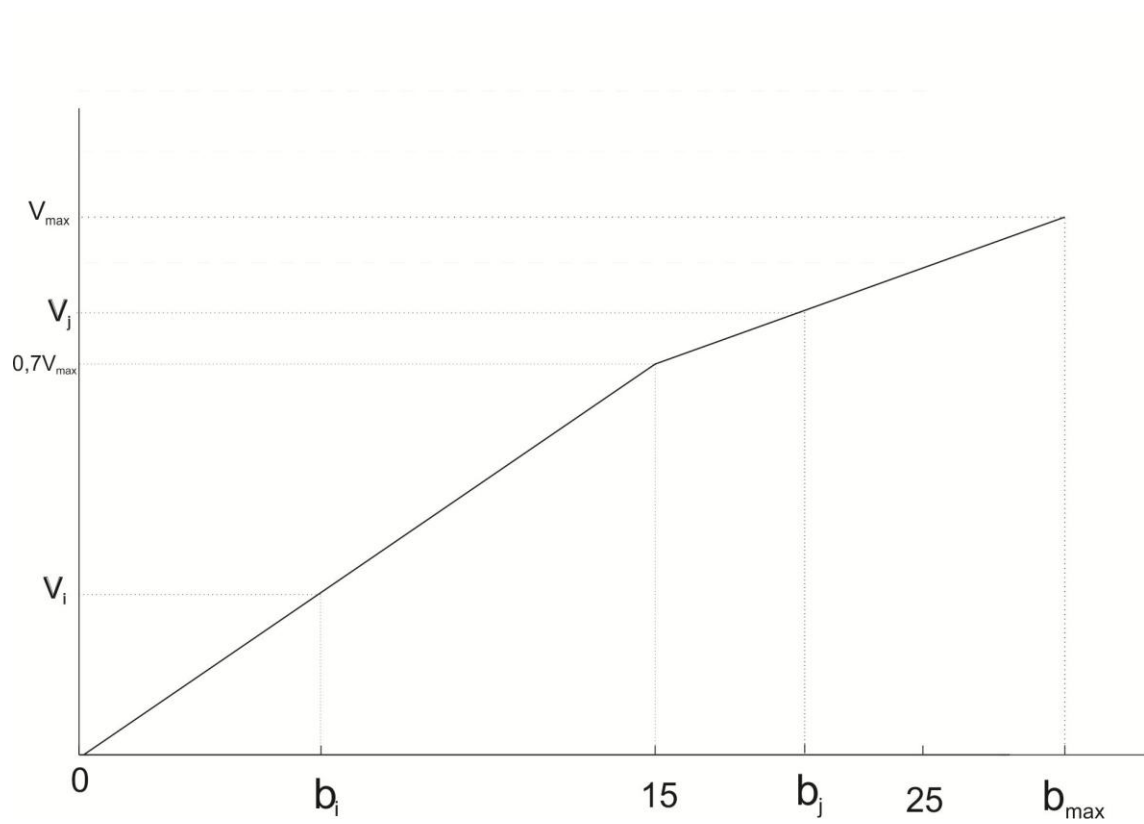
Figura 3: Representación gráfica das puntuaciones se b_{\max} \geq 25 .
