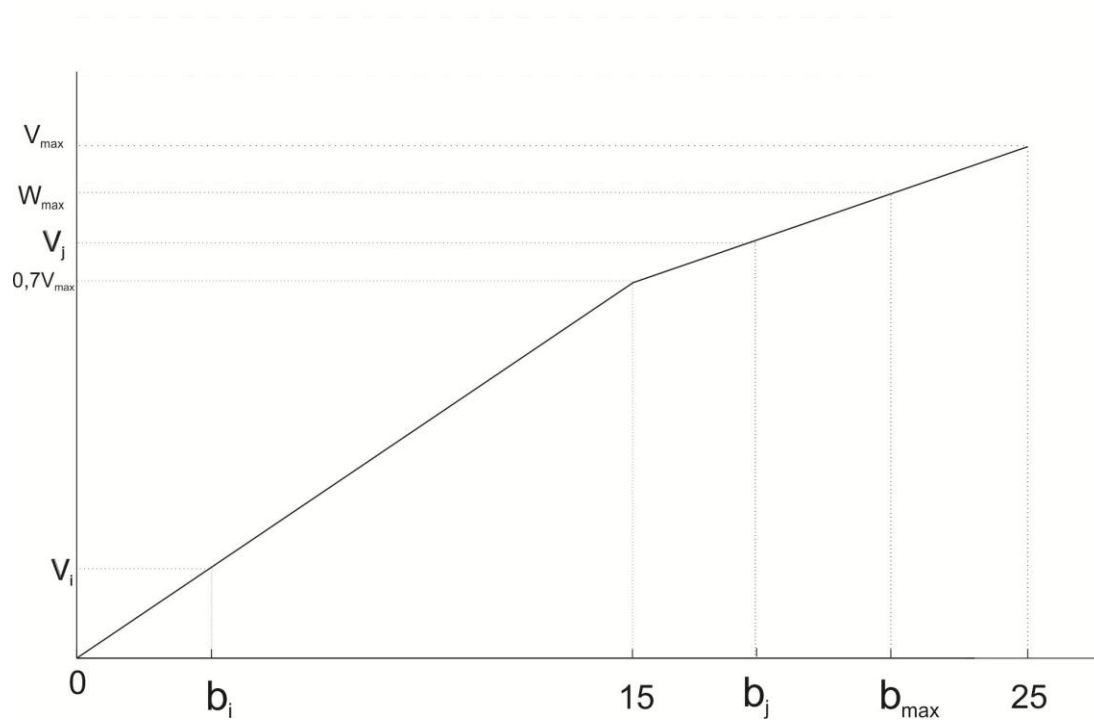
Figura 2: Representación gráfica de las puntuaciones si 15 \leq b_{max} < 25 .
