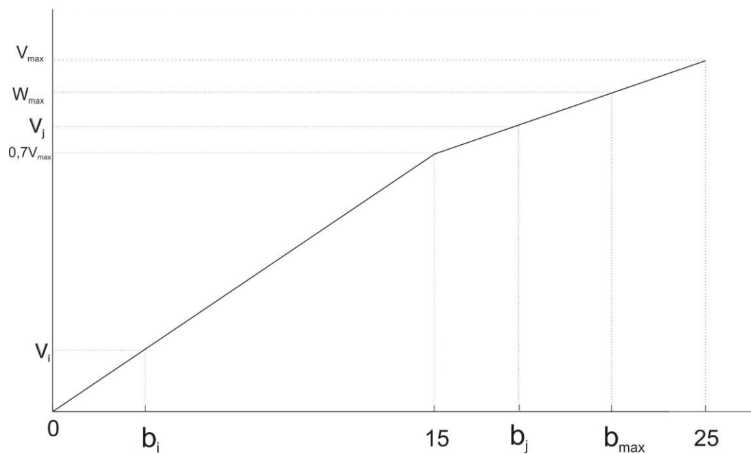
Figura 2: Representación gráfica das puntuaciónes se 15 \leq b_{\max} < 25 .
