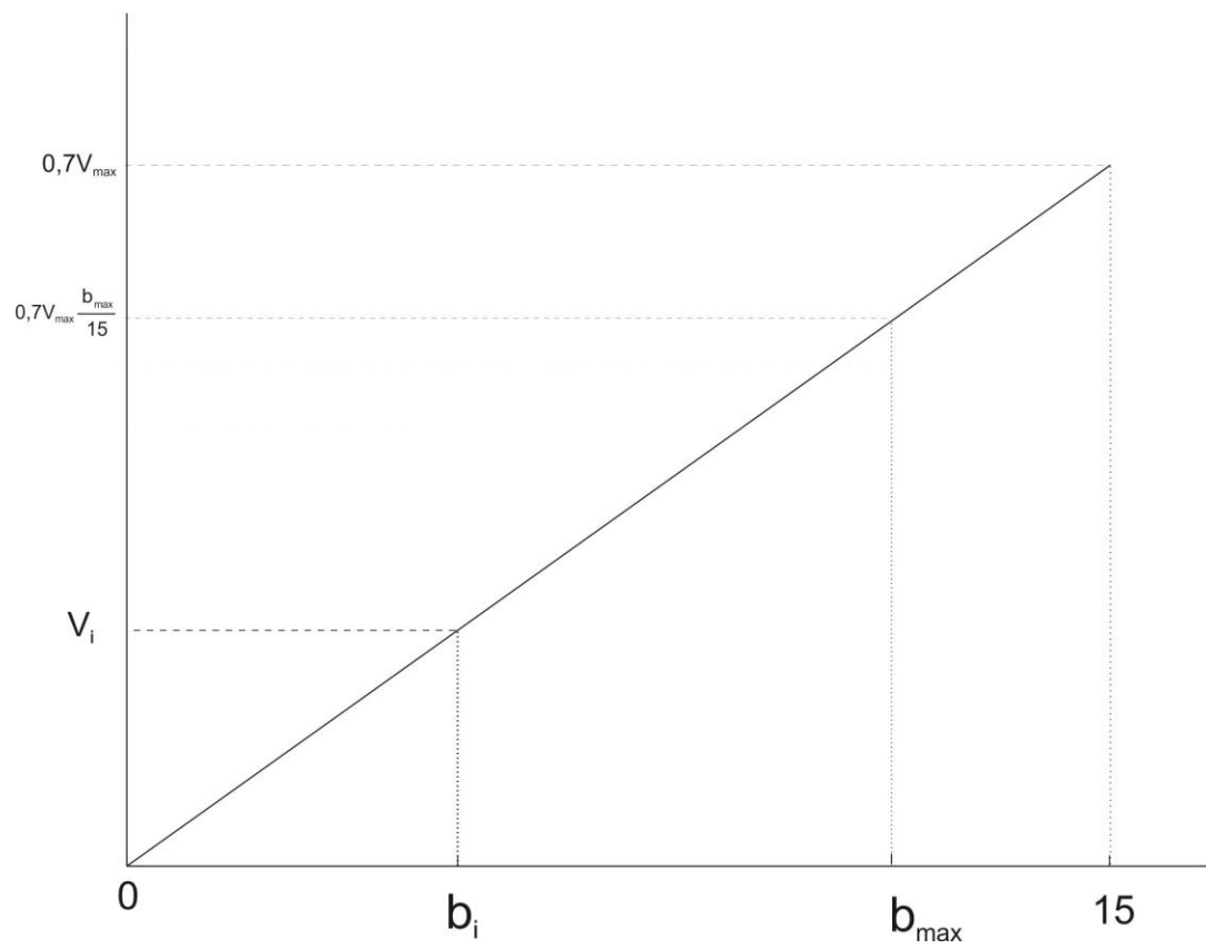
Figura 1: Representación gráfica de las puntuaciones si b_{\max} < 15 .
