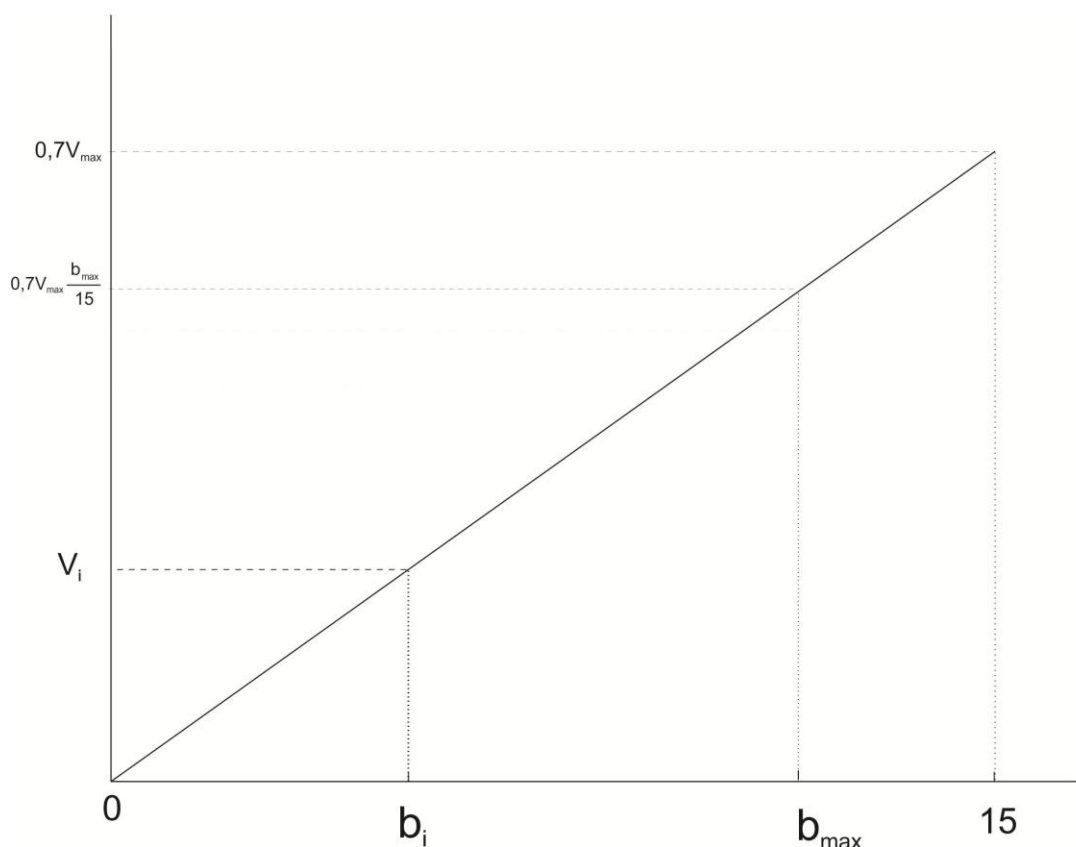
Figura 1: Representación gráfica das puntuaciones se b_{\max} < 15 .
