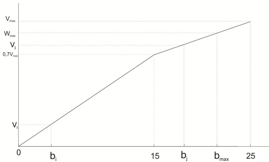
Figura 2: Representación gráfica de las puntuaciones si 15 \leq b_{\max} < 25 .
