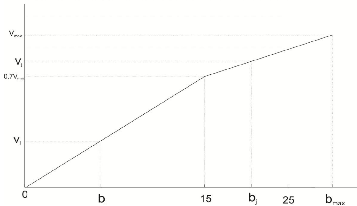
Figura 3: Representación gráfica de las puntuaciones si b_{\max} \geq 25 .
